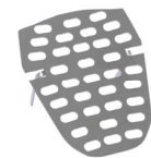
SLA 26
