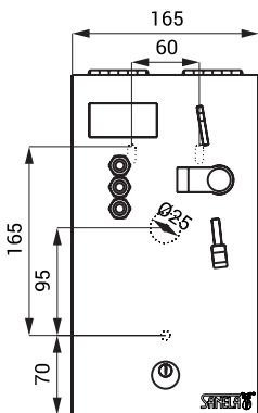
SLZA 01LN
