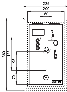
SLZA 01LNZ
